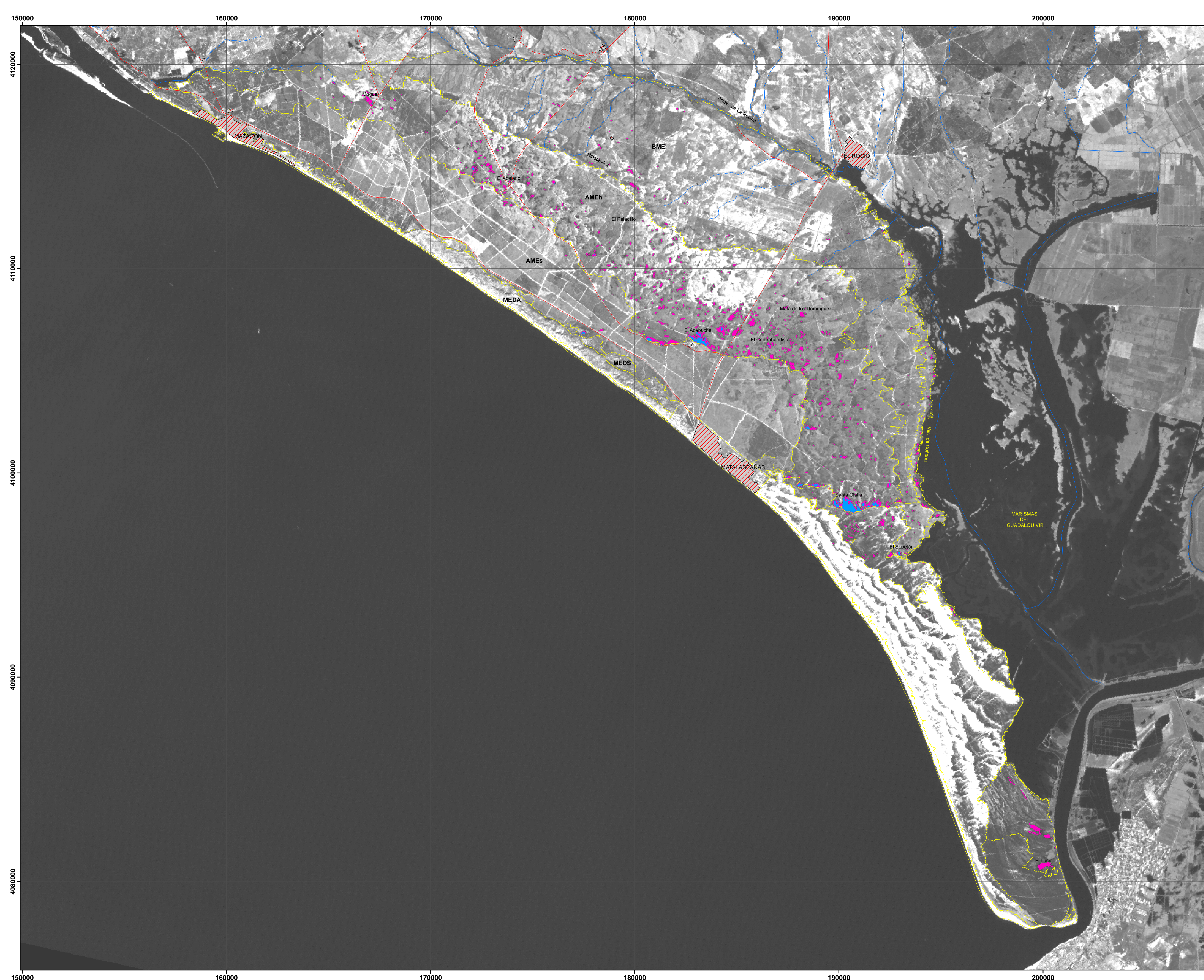
Cartografía de lámina de agua y superficies encharcadas. Marzo 1998. Landsat TM
